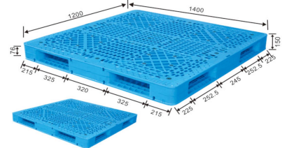
ENL-H1412WSD 140 x 120 x 15 cm
