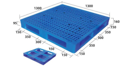
ENL-1313C 130 x 130 x 16 cm
