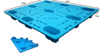
ENL-1210CS 120 x 100 x 15 cm
