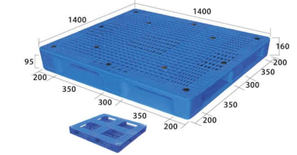
ENL-1414C 140 x 140 x 16 cm
