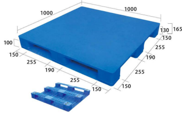
ENL-1010H 100 x 100 x 16.5 cm
