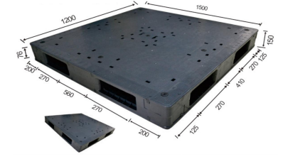
ENL-H1512PSB 150 x 120 x 15 cm
