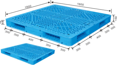
ENL-1616WSA 160 x 160 x 15 cm
