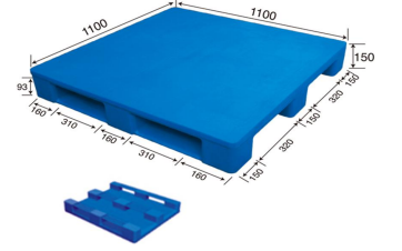
ENL-1111PGC 110 x 110 x 15 cm
